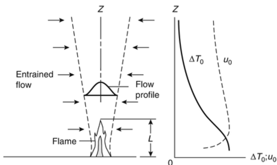
Figure 54 : Vue schématique d'un panache d'incendie et grandeurs thermocinétiques, selon [91]
