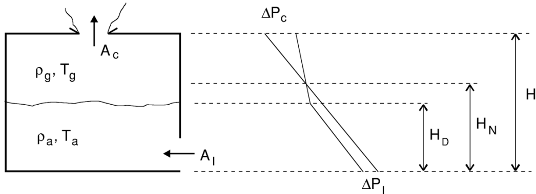
Figure 59 : Représentation schématique d'un incendie confiné, selon [94]
