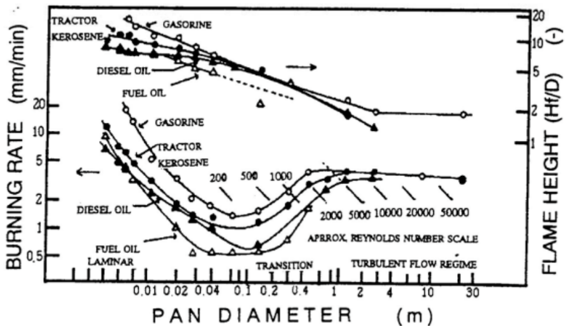
Figure 33 : Evolution de la vitesse de combustion selon la taille du foyer pour des combustibles liquides, d'après [81]
