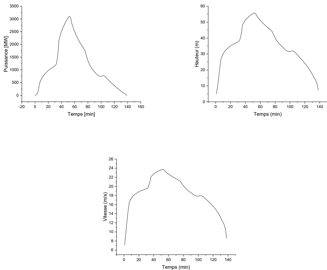
Figure 57 : Courbe de puissance et caractéristiques du panache estimées pour l'incendie sur site Allopneu
