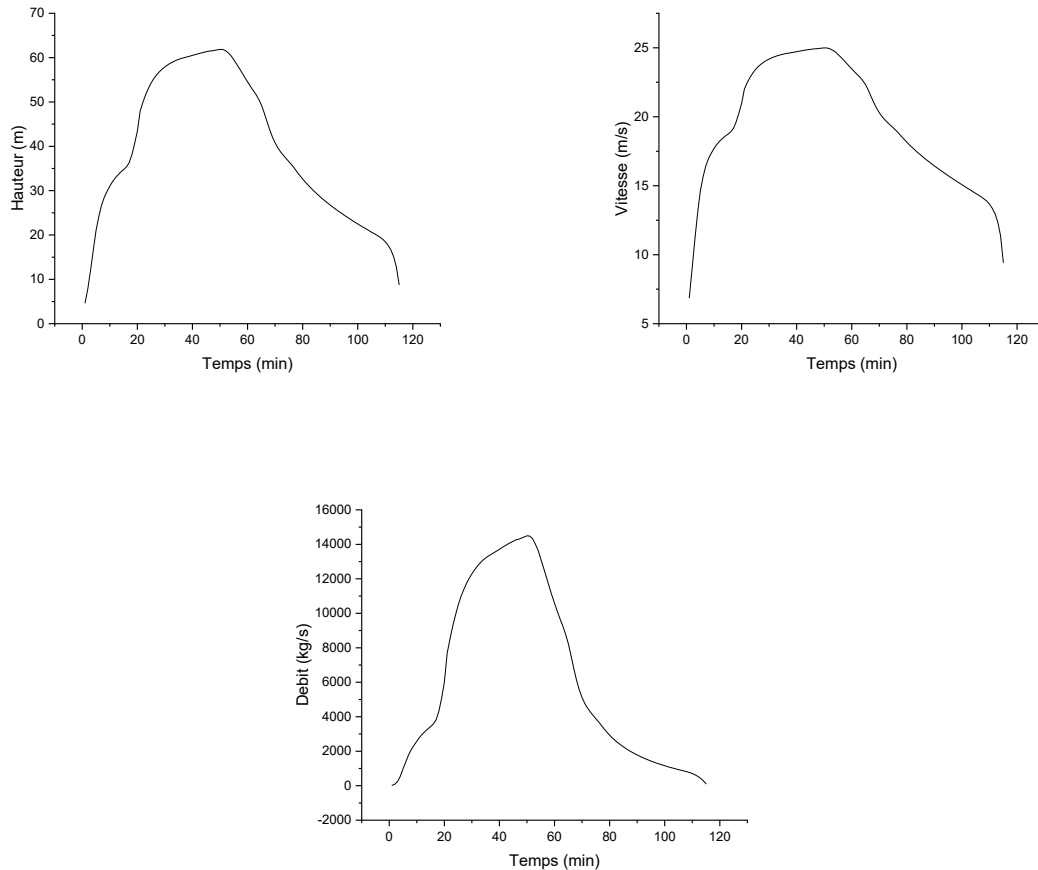
Figure 56 : Evolution des caractéristiques du panache au cours du temps
