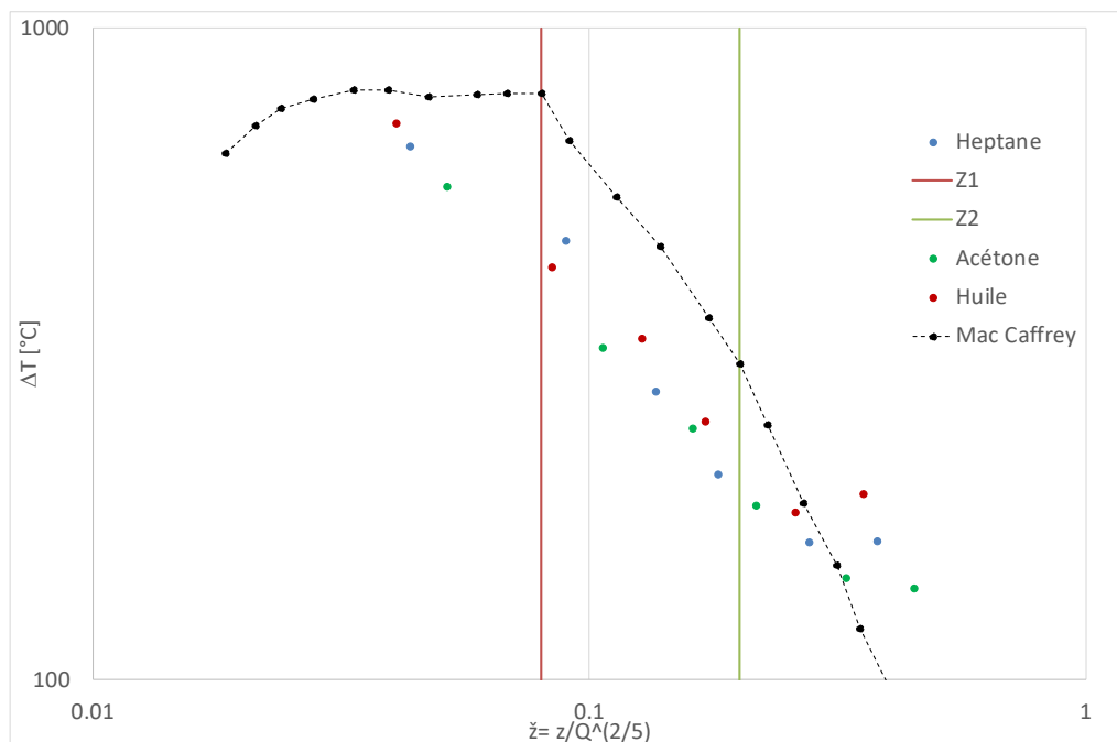
Figure 34 : Profil vertical adimensionné de température pour les feux de nappe d'acétone ( 0,25 \text{ m}^2 ), d'heptane ( 0,25 \text{ m}^2 ) et d'huile ( 0,5 \text{ m}^2 )
