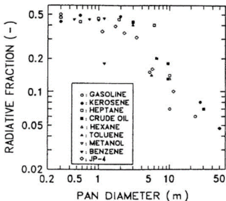
Figure 31 : Evolution de la fraction radiative en fonction du diamètre caractéristique du foyer, selon [80]
