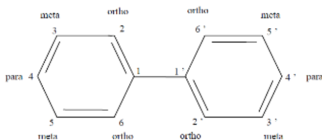
Figure 15 : Structure moléculaire des PCB
