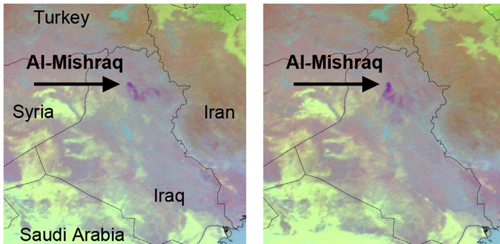
Figure 7 : Image du satellite SIVIRI lors du feu de soufre d'Al-Mishraq, selon [19]
