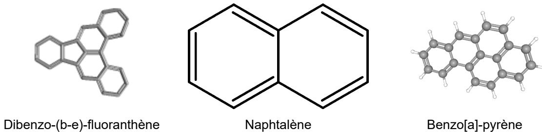
Figure 13 : Exemple des HAP
