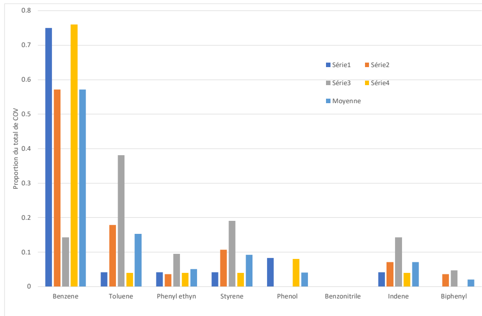
Figure 26 : Proportion de COV lors du brulage de pneumatiques, selon [71]
