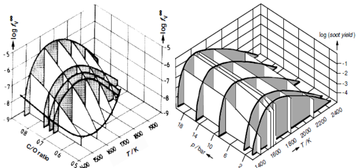
Figure 12 : Evolution du taux volumique de suies en fonction de la température, du rapport C/O et de la pression, selon [37]
